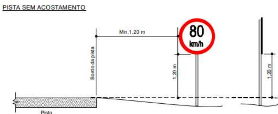
Figura 5 – Posicionamento dos sinais de regulamentação – Pista sem acostamento
