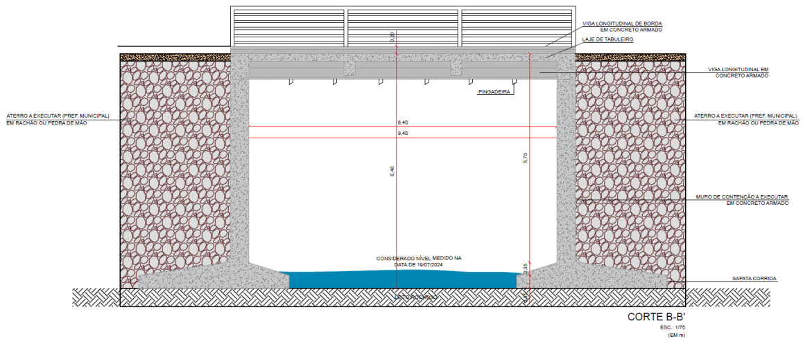
Figura 2 - perfil longitudinal da ponte projetada
