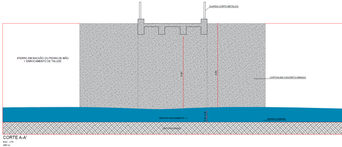
Figura 1 - Seção transversal projetada
