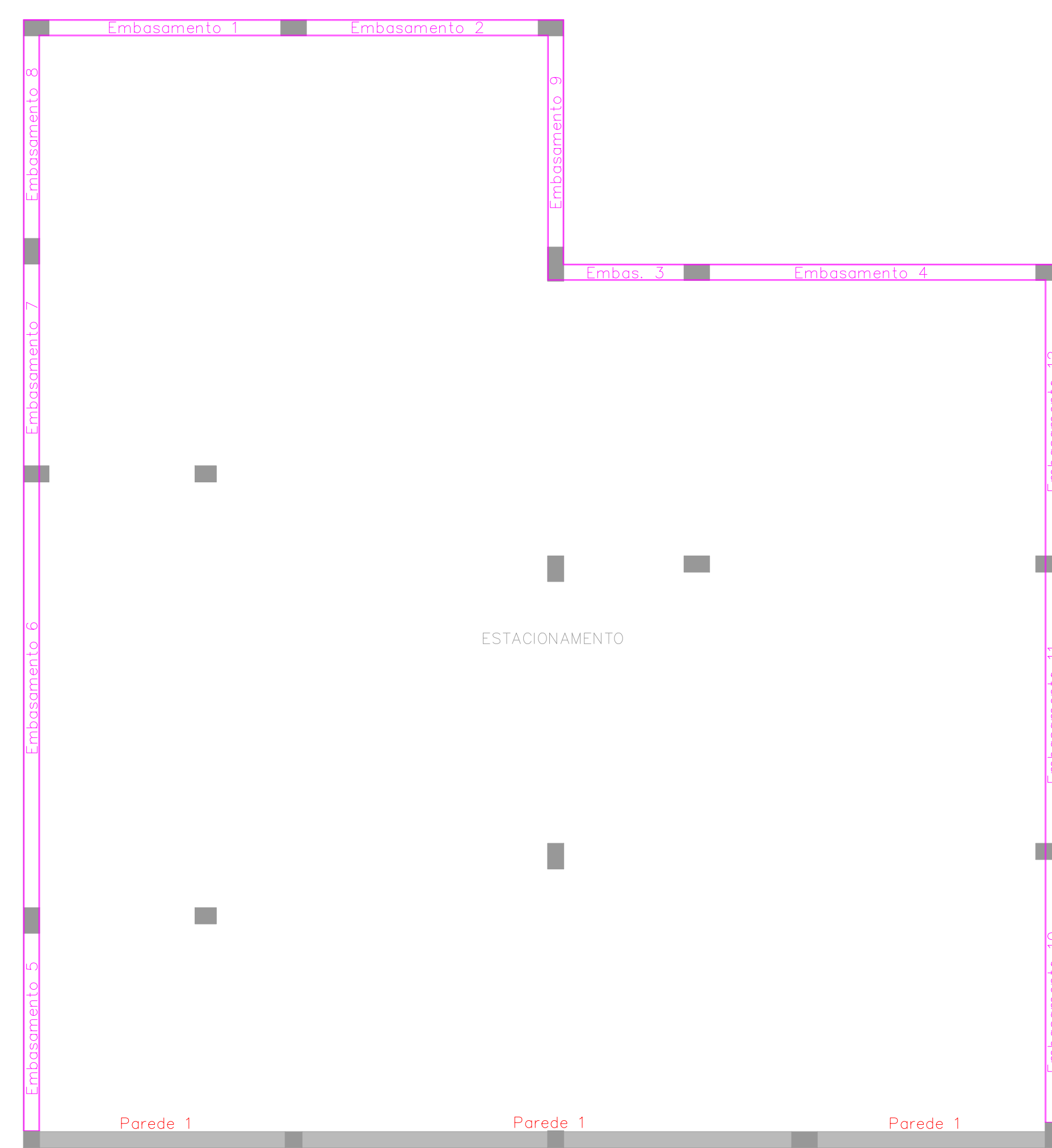
Planta Paredes Baldrame Escala.....1/50
