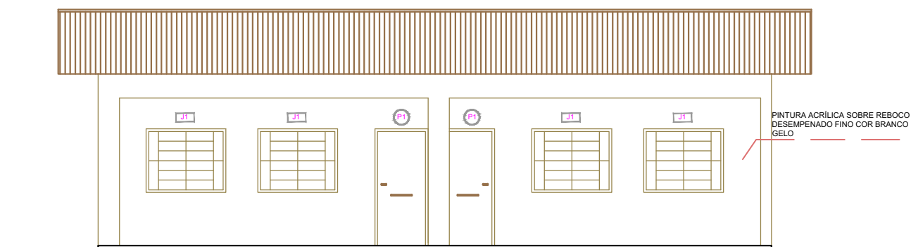
FACHADA SUL ESCALA.....1/100
