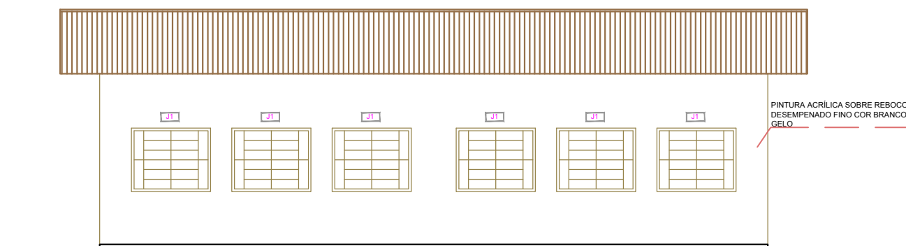
FACHADA NORTE ESCALA.....1/100
