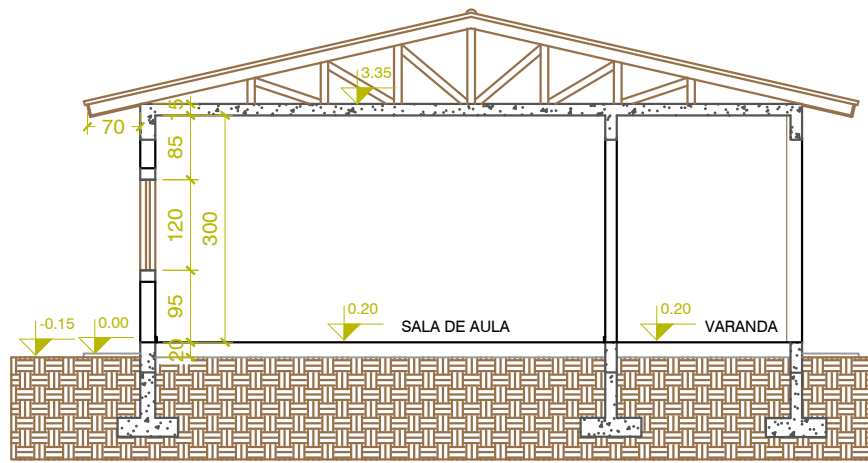
CORTE B-B ESCALA.....1/100
