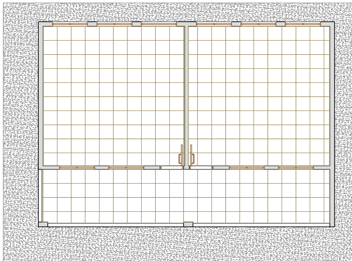
PLANTA PAGINAÇÃO ESCALA.....1/100
