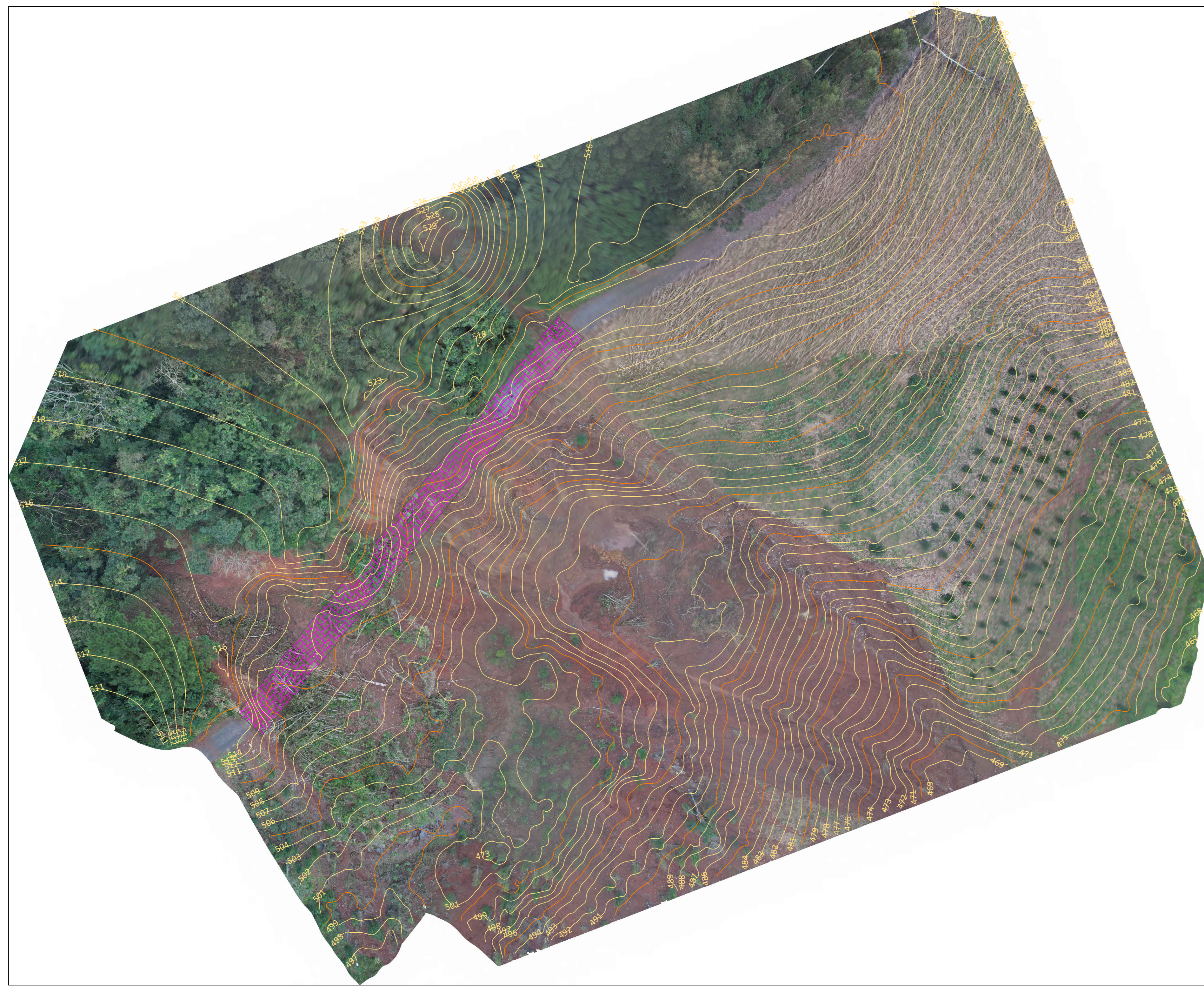
PLANTA PLANALTIMÉTRICA ESC.: 1/500 (EM m)
