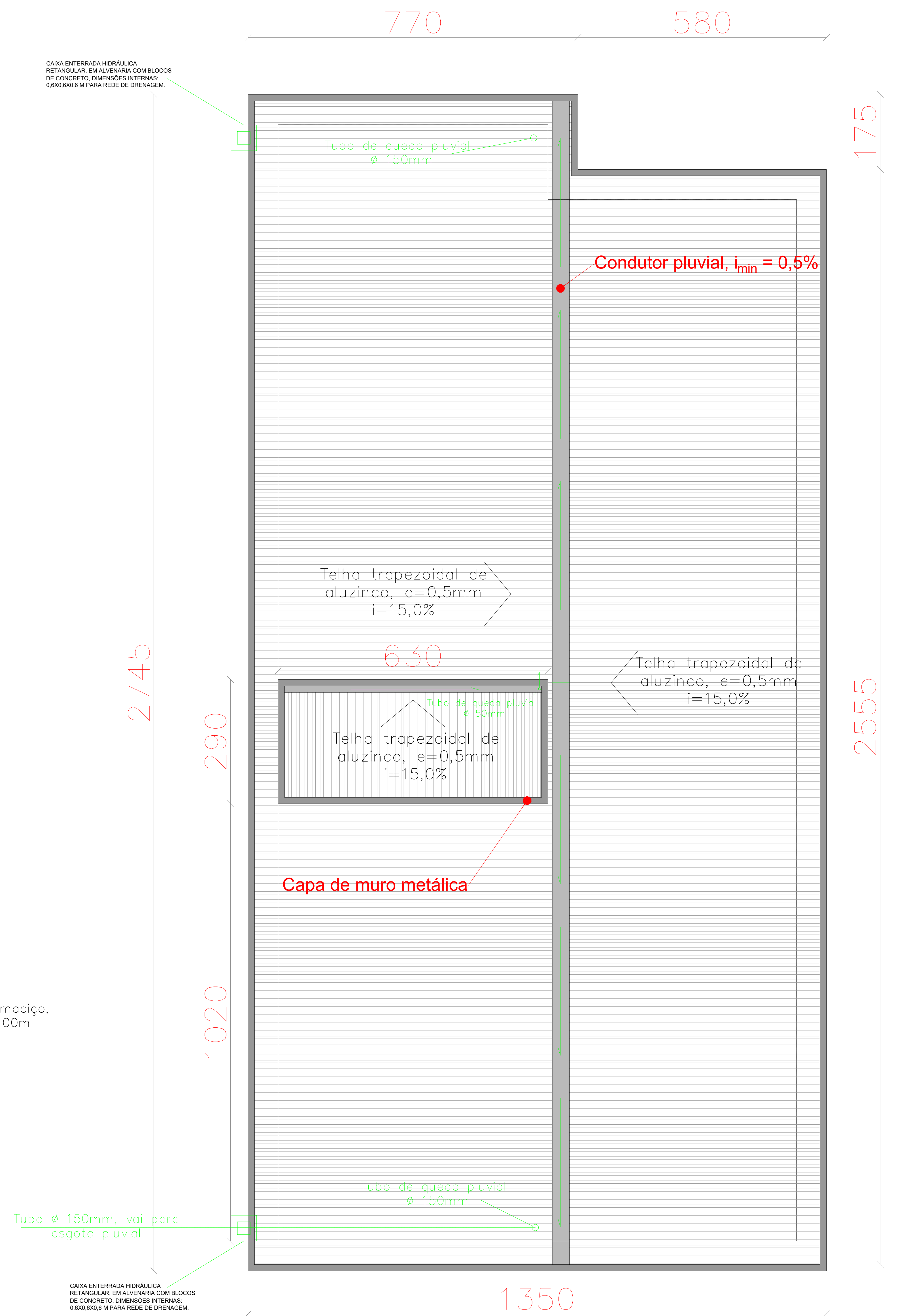
Planta Baixa Cobertura Escala.....1/50
